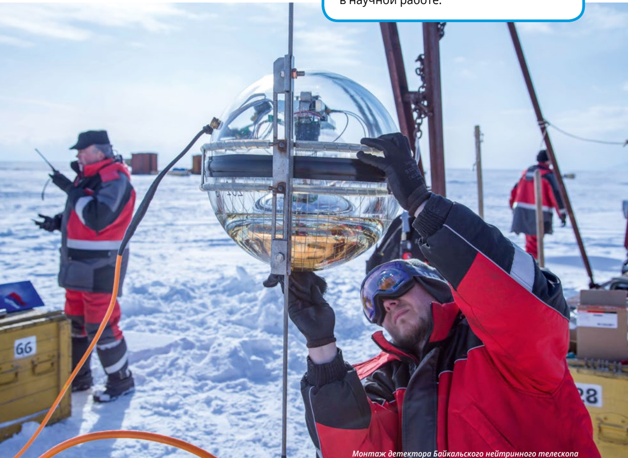
Монтаж детектора Байкальского нейтринного телескопа
